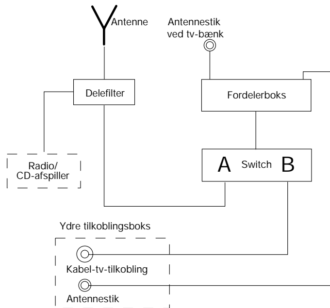
Skema over antennesystem
