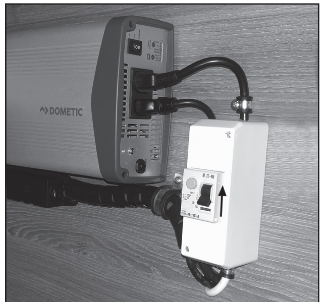
Bij de inverter is een aardlekschakelaar gemonteerd.
