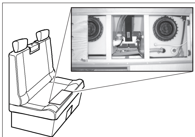
Tuorevesisäiliön tyhjennys.
