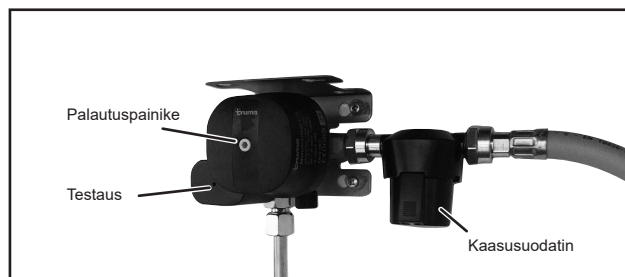
Truma MonoControl on tarkoitettu yhdelle nestekaasupullolle.
