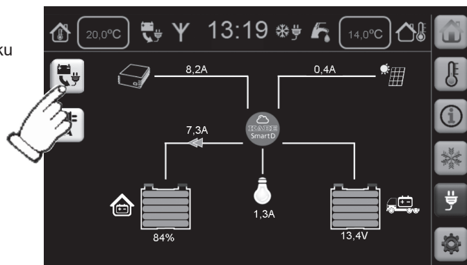
Käynnistä ja sulje invertteri ohjauspaneelistä.
