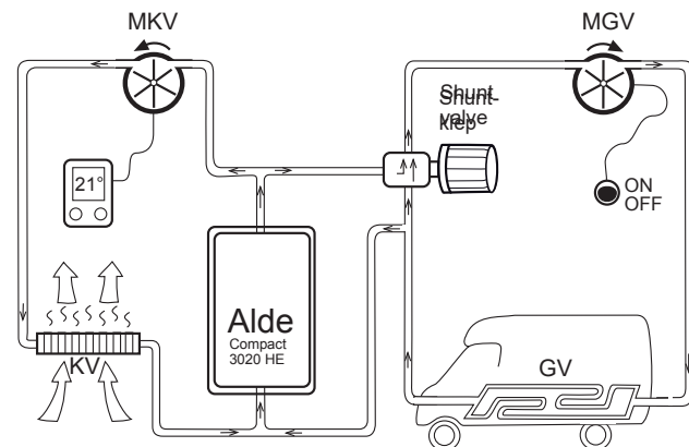
Figuur 2: Schematische illustratie van het verwarmingssysteem AGS II Pro van het woongedeelte (vloerverwarming met shuntklep).
