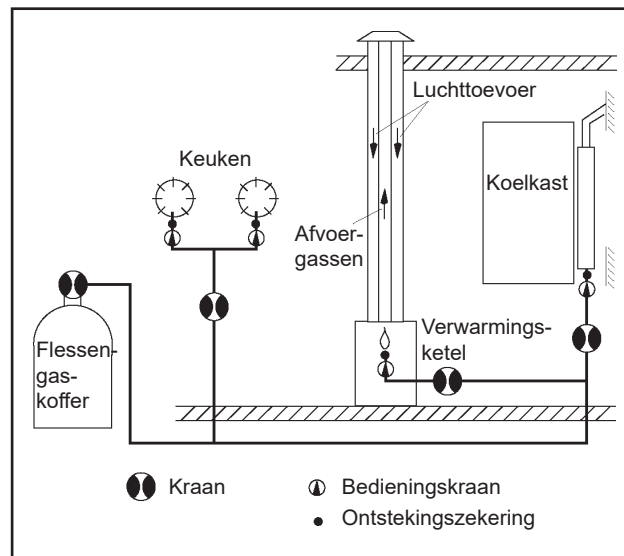
Schematische afbeelding van het flessengassysteem
