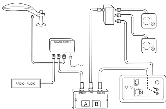
Schematisk illustration av antenssystemet.
