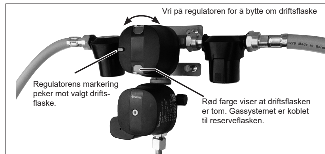
Truma DuoControl er beregnet på to gassflasker.
