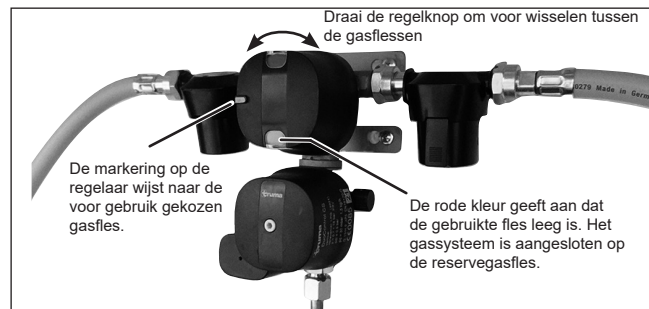
Truma DuoControl is ontworpen voor twee gasflessen.
