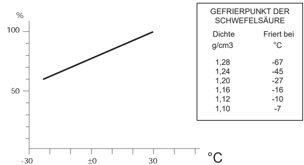
Leistung der Batterie bei verschiedenen Temperaturen.
