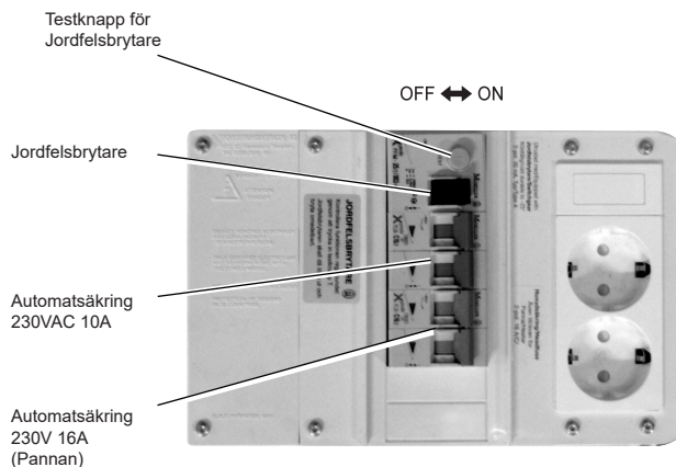
Elboxens baksida
