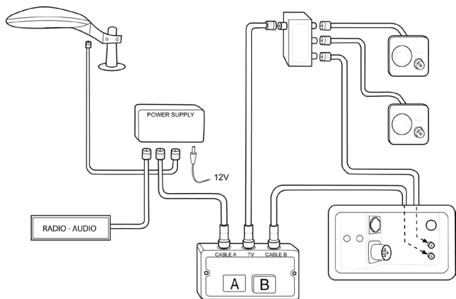
Kaaviokuva antennijärjestelmästä.
