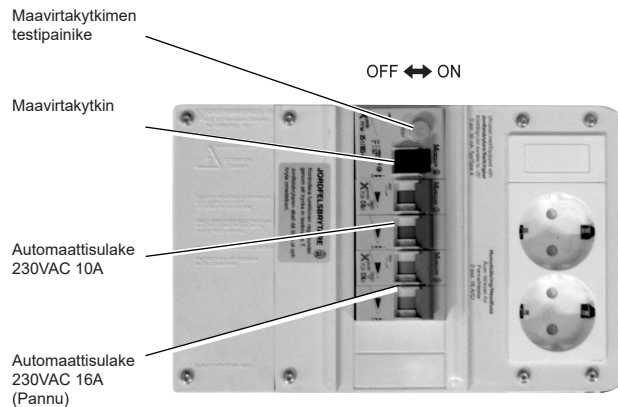
Sähkökotelon takaosa
