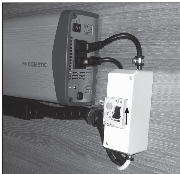
Ein Erdschluss-Schalter ist am Spannungswandler montiert.
