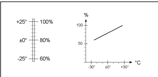
Batteriekapazität bei unterschiedlichen Temperaturen.
