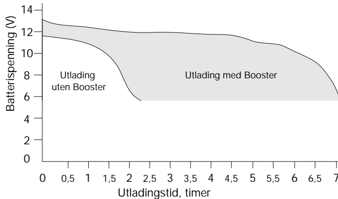
Utladningsforløp med 100 W belastning, batteri 65 Ah Panasonic LCL12V65P (gelétype)
