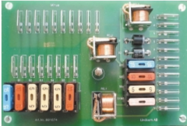
Piirikortissa
