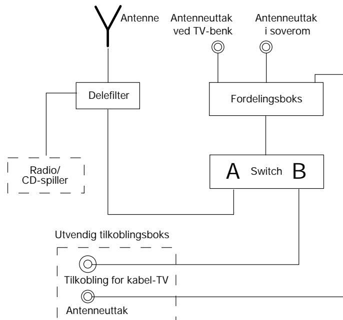
Skjema over antennesystem
