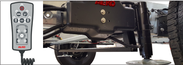
AL-KO HY4 hydrauliska stödben. Ställ bilen i våg med ett enda knapptryck på handkontrollen. Ett nytt knapptryck och så är sängläge med en liten lutning framåt inställt. Ännu ett knapptryck och benen åker helt in. HY4 kan även köras helt manuellt där man kan styra kombinationer av stödbenspar så som man önskar. Varje ben har en egen motor och hela systemet är monterat på chassit. Inga oljeslangar dras inne i bilen. HY4 är standard på Imperial, tillval på övriga.
