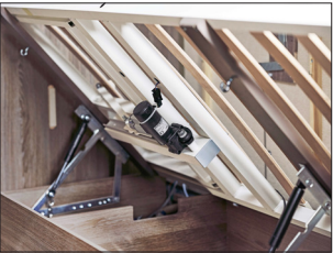
Elektrisk huvudgärde säng (standard Imperial LT och LQB modeller). Vid tillvalet minskar garagehöjden med 10 cm.
