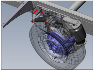
AL-KO 2-kanals luftfjädring (ej Novum Compact)
