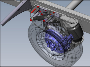
AL-KO 2-kanals luftaffjedring (ikke Novum Compact)
