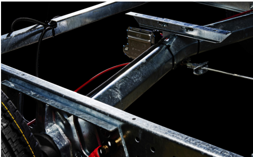
Chassis med ekstra vridstivhed. Ekstra tværvange mellem langsgående vanger giver et mere stabilt gulv og et chassis med ekstra vridstivhed. Tværvanger for bedste stabilitet. Chassiset har udliggere fra den længdeforløbende sidevange som aflastning for vægten, hvor gulv og væg er samlet. Karosseriet kan tåle en meget høj belastning, for eksempel når der ligger store mængder sne på taget.
