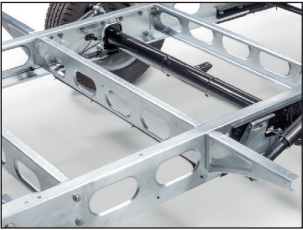
Chassis pakket 4250 kg Chassis pakket 4400 kg (met 180 pk motor)
