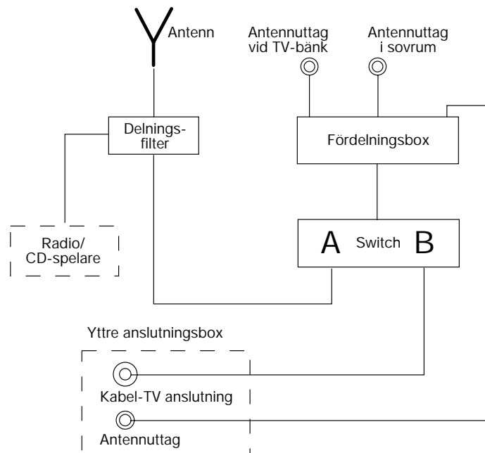
Schema antensystem
