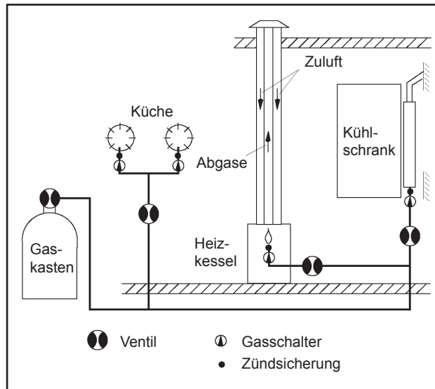
Schematische Darstellung des Gasversorgungssystems.
