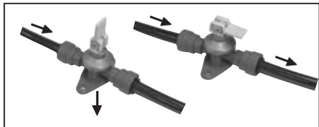
Ablasshahn für den Boiler. Offene bzw. geschlossene Stellung.
