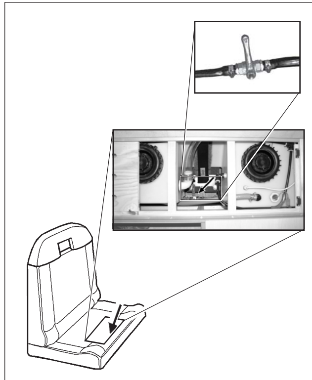
Vattensystemets avtappningskran för färskvatten.
