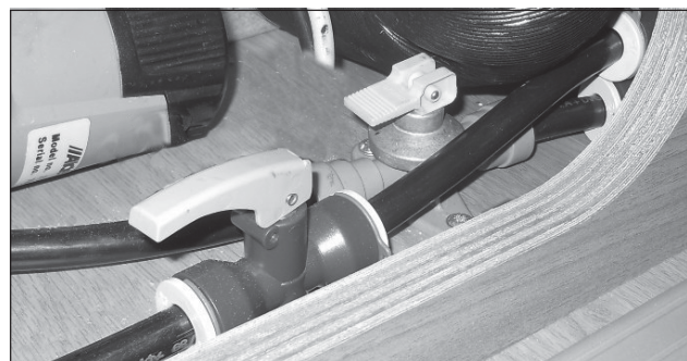
Avtappningskranar för kall- och varmvattenslang.
