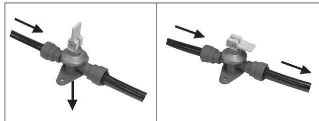
Avtappningsventil för varmvattenberedaren. Öppet respektive stängt läge.
