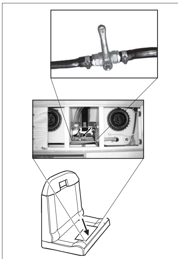
Der Frischwasser-Ablasshahn des Wassersystems.
