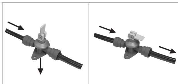
Ablasshahn für den Boiler. Offene bzw. geschlossene Stellung.
