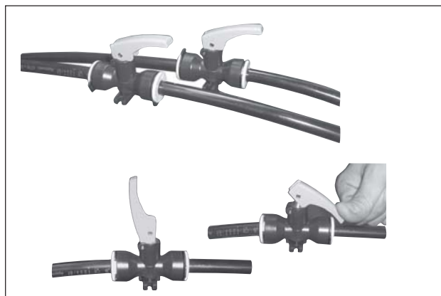
Ablasshähne für Kalt- und Warmwasserschläuche.
