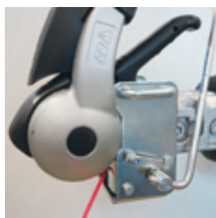
Puller Winch (X0204) Smart spil til sikker opkobling, beregnet til at blive monteret på kuglekobling og manøvreres ved hjælp af udtageligt håndtag
