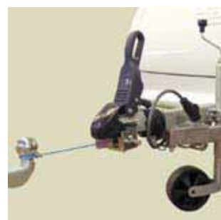
Puller Winch Treklier (X0204) Voor veilige koppeling. De Puller Winch past op de meeste kogelkoppelingen en wordt bediend met een stang met 17 mm dop.
