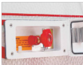
Uitwendige gasaansluiting Voor aansluiting van barbecue buiten de caravan.
