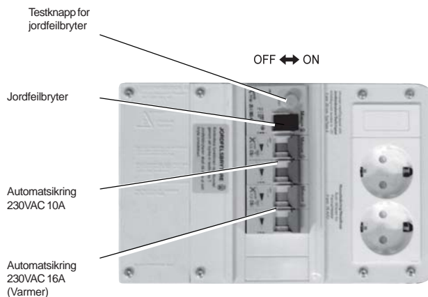
Elboksens bakside
