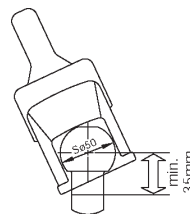
Kuglehals, trækkøretøj
