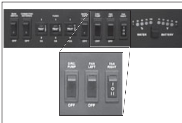
Lämpöpaketin kytkin ohjauspaneelissa.
