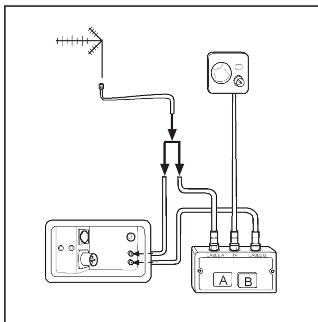
Matkailuauton antennijärjestelmän kytkentäkaavio,
