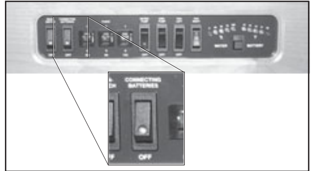
Katkaisija "CONNECTING BATTERIES", jolla yhdistetään asunto-osan ja auton 12V-järjestelmät.
