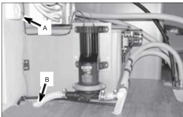
Harmaavesisäiliön tyhjennuspumppu kytkimiseen (A) ja poistoletkuineen (B).
