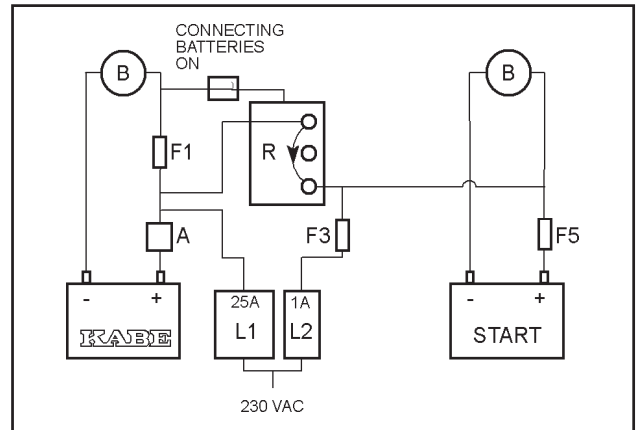
Kaavio asunto-osan akun käynnistysavusta auton akulle. B kuvaa muita sähkökuormia vastaavissa järjestelmissä. R kuvaa latausvirran jakajaa. L kuvaa akkukurilla.
