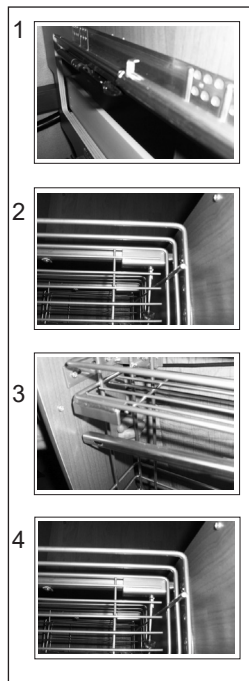
Auszugfach montieren
