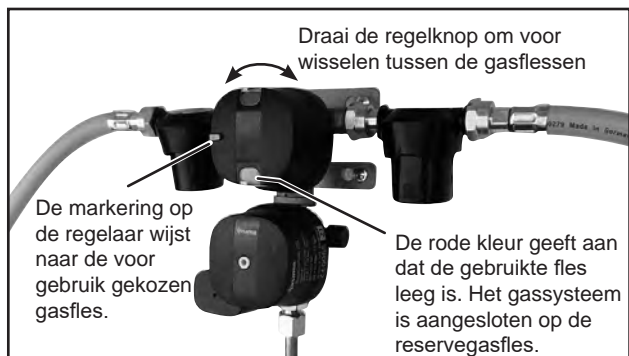
Truma DuoControl is ontworpen voor twee gasflessen.
