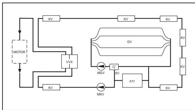
Halfgeïntegreerde camper met AGS II Pro (met shuntklep).
