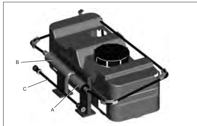
Vandrensningsehederne er monteret ved friskvandstanken.
