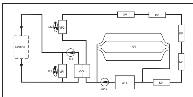
Halvintegret bil.
