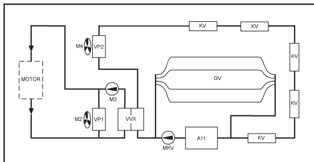
Halvintegrrert bobil.
