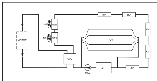
Helintegret bil.
