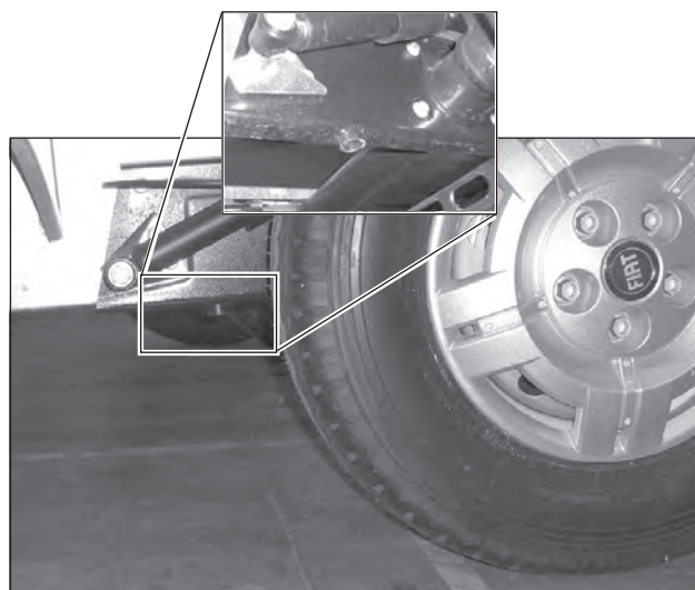
Kriksteunpunt
