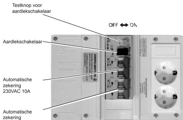
Achterzijde van de elektriciteitscentrale
