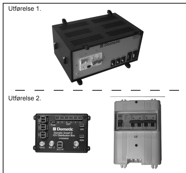
Den elektriske sentralenheten.
