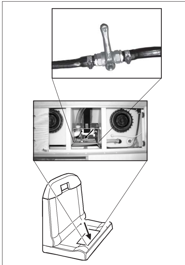
Vesijärjestelmän tuoreveden tyhjennyshana.
