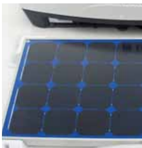
Solcellpanel Y0163 85 W inkl. regulator och övervakningspanel.
