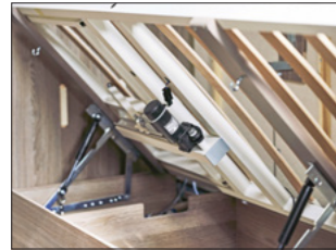
Elektrisk hev- og senkbar hodeende (standard Imperial og LQB-modeller)
