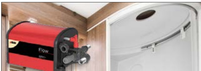
Alde Flow. Met Alde Flow kunt u warm douchen zolang u maar wilt! Alde Flow is een aparte warmwatertank die wordt aangesloten op het glycolverwarmingssysteem. De tank verwarmt vers water voordat het de gewone warmwatertank van de verwarmingsketel bereikt en zorgt voor permanent warm water in de kranen.
