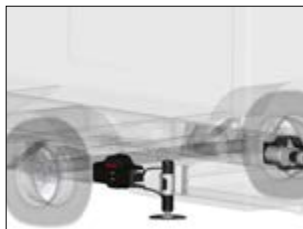
Hydraulische Ausdrehstützen (standard Imperial)
