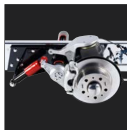
Luftfjæring AL-KO 780, i760, i810 X2 tvåksel 880, i860, i910 X2 treaksel i810 Tandem X2 treaksel
