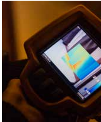
Mit Hilfe von Wärmekameras stellen wir sicher, dass unsere Konstruktion genau der Qualität entspricht, die wir anstreben.
