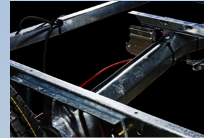
Ekstra vridningsstivt chassis. Ekstra bjelker mellom langsgående chassisrammer gir mer stabilt gulv og ekstra vridningsstivt chassis. Mellombjelker for beste stabilitet. Chassiset har utstikkere fra langsgående sidebjelke for å avlaste tyngden der gulv og vegg er sammenføyd. Karosseriet tåler veldig høy belastning, for eksempel når store mengder snø ligger på taket.
