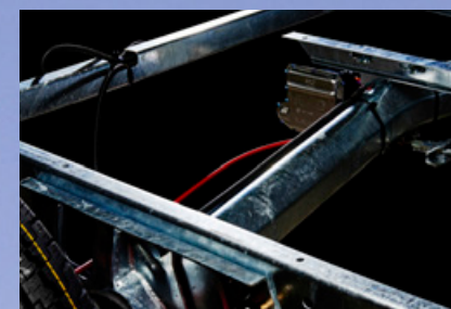
Ekstra vridningsstivt chassis. Ekstra bjelker mellom langsgående chassisrammer gir stabilere gulv og ekstra vridningsstivt chassis. Mellombjelker for beste stabilitet. Chassiset har utstikkere fra langsgående sidebjelke for å avlaste tyngden der gulv og vegg er sammenføyd. Karosseriet tåler veldig høy belastning, for eksempel når store mengder snø ligger på taket.
