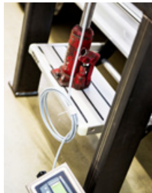
Painetta käytetään tuotteiden lujuuden testaukseen.
