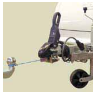
Puller Winch (X0204) For sikker tilkopleing. Puller Winch passer til de fleste kulekoplinger og betjenes ved hjelp av sperreskaft med 17 mm pipe.
