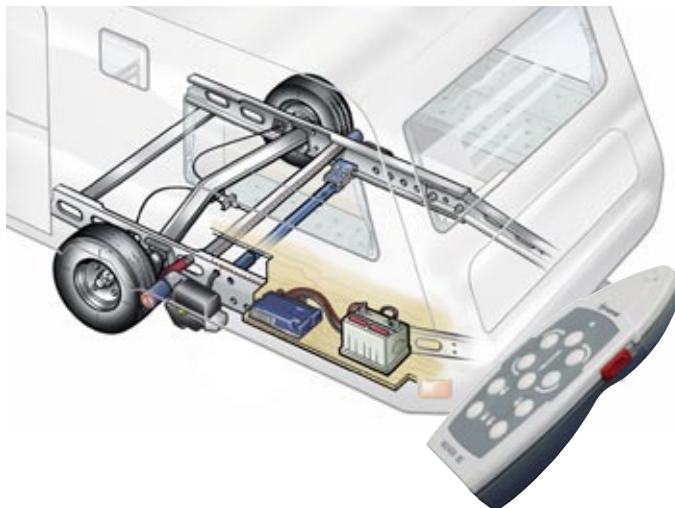
TRUMA Move Control: Tandemachse X0216 Einzelachse X0217
