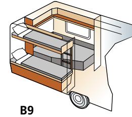
B9 B 196 x 140/118 + 2 x 196 x 68
