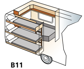
B11 B 196 x 140/118 + 2 x 196 x 68 + 1 x 196 x 62
