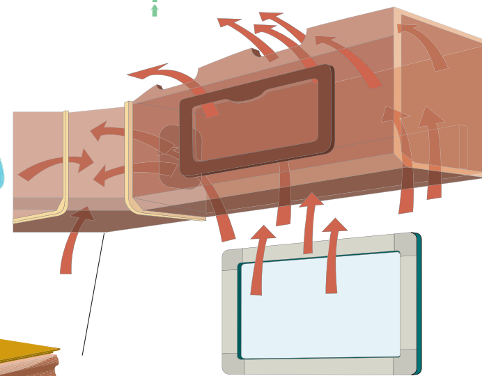
Ovanskåpen med sina ventilationsöppningar och luftkanaler som gör att den varma luften kan cirkulera obehindrat genom skåpen – även när de är fulla med kläder – och tillbaka in mot mitten av fordonet.
