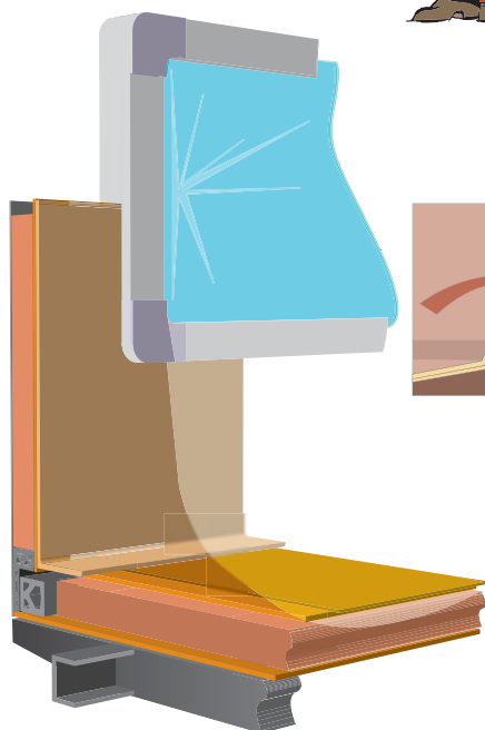
Den kraftiga isoleringen gör att husvagnen håller sig sval om sommaren och varm på vintern. I hela konstruktionen använder vi Ecoprimsolering – en isolering som är tillverkad med slutna celler, vilket gör att den inte kan ta åt sig någon fukt.
