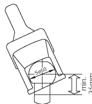
Kogelhals trekauto
