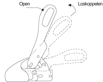
Loskoppelen
